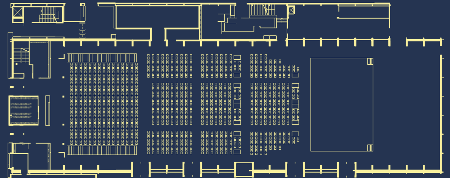
CONGRÈS GRANDE JAUGE / 1431 places / dont 20 places PMR
